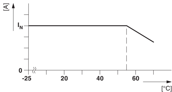
Bild 10 Temperature-dependent derating
