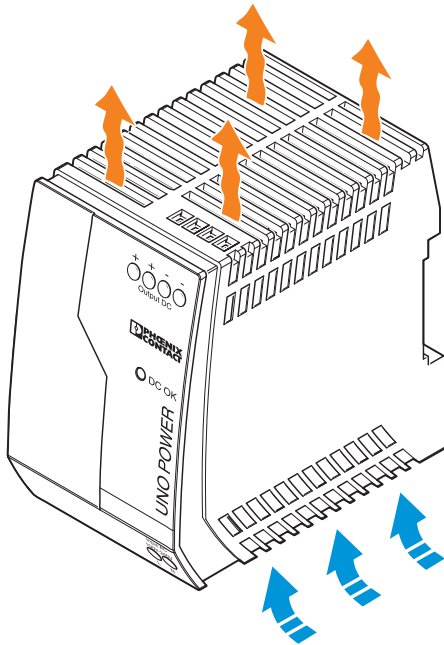
Bild 2 Convection
